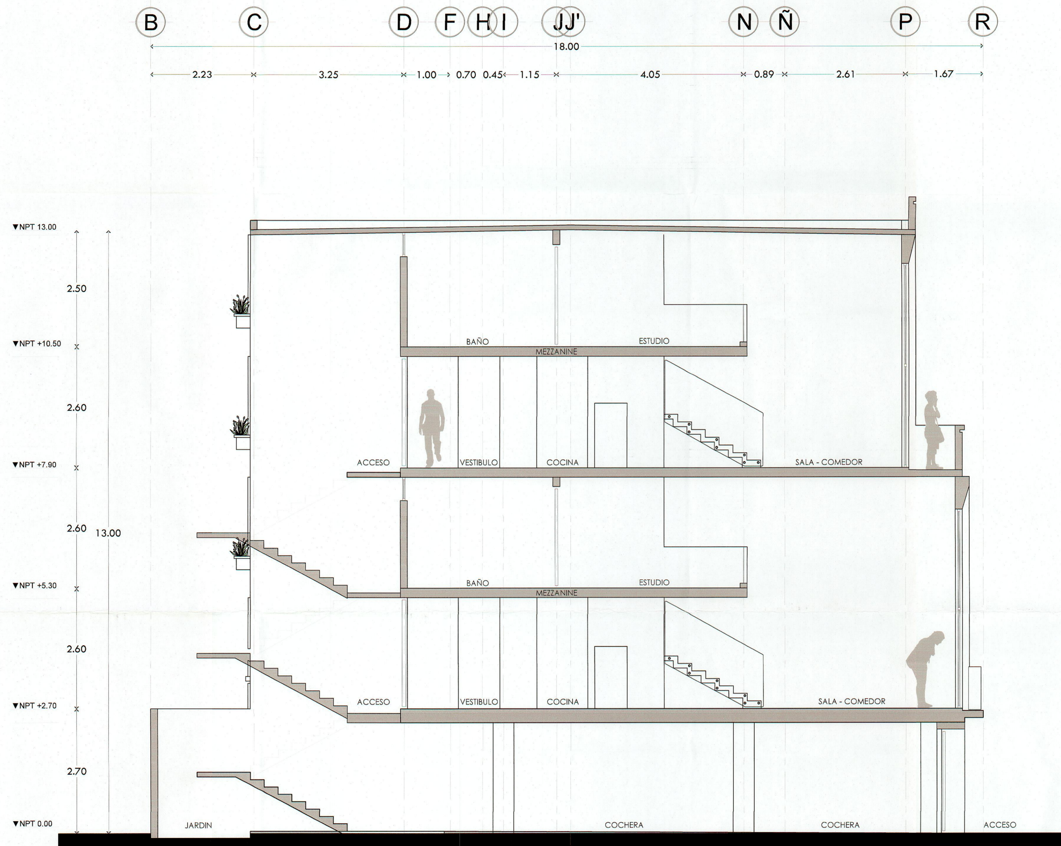
Corte A-A' Arquitectónico
