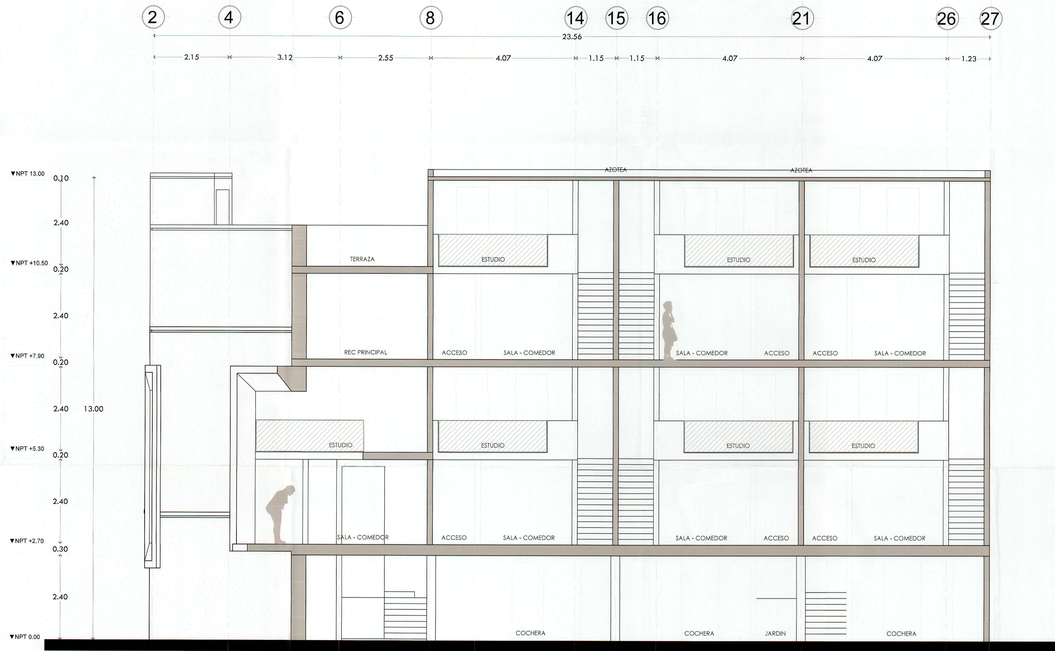
Corte B-B' Arquitectónico
